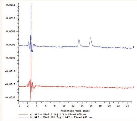
圖五、高效液相層析圖譜
