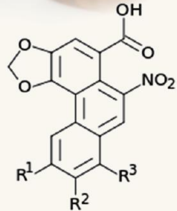
圖一、馬兜鈴酸 I R1: -H, R2: -H R3: -OCH3 馬兜鈴酸 II R1: -H, R2: -H R3: -H
